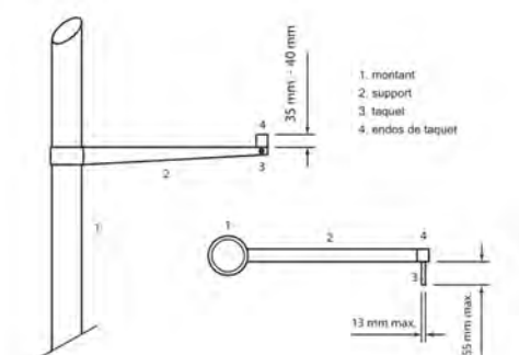
Schéma (b) RT28 – Support de barre transversale (vue de la zone de réception et vue en plan)
